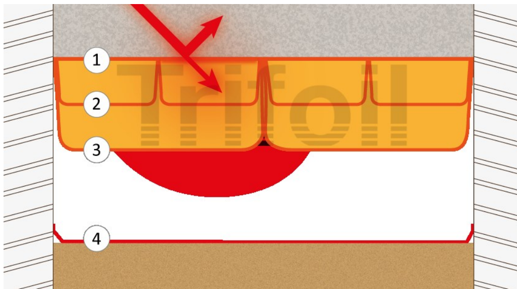
Trifoil isolatiekussens (1,2,3) met bodemfolie (4)
